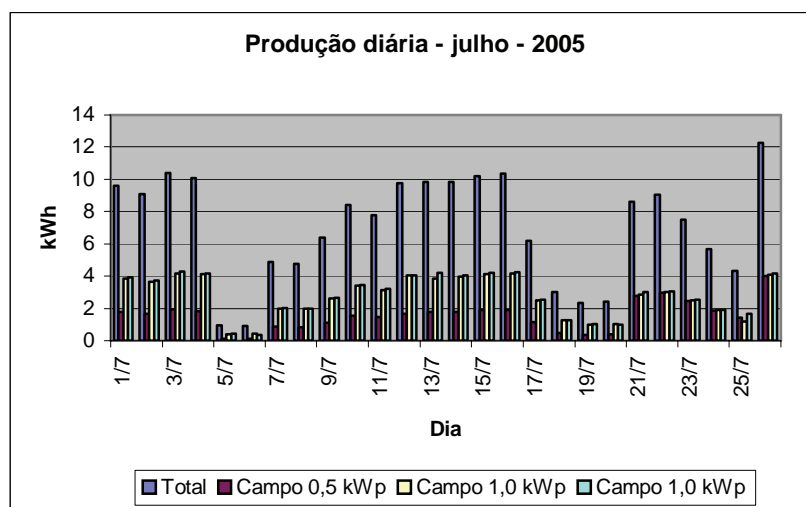
Figura 26. Produção diária de energia elétrica do sistema de 2,5 kWp, mês julho.
