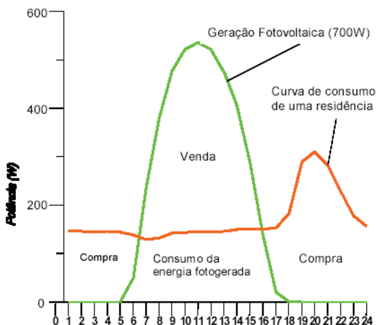
Figura 3. Curva de carga de uma residência (em vermelho), contrastada com a curva de produção de um sistema fotovoltaico com 700 Wp instalados (em verde).
