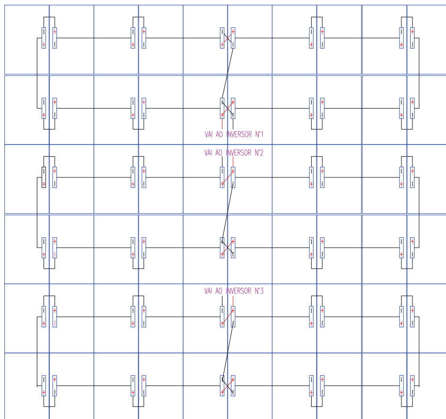
Figura 15. Configuração das conexões.
