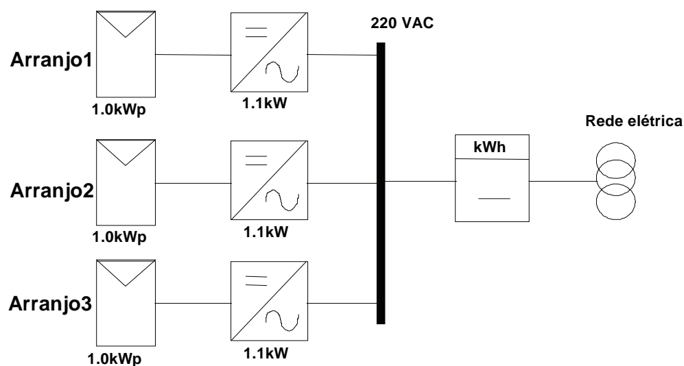
Figura 13. Diagrama unifilar do sistema.
