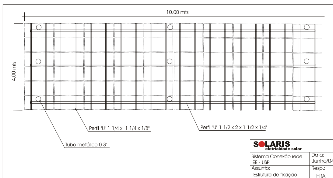
Figura 11. Esquema de sustentação
