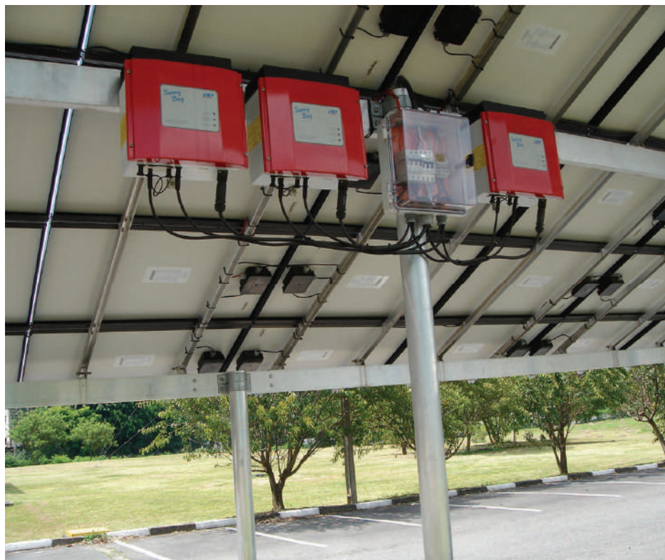
Figura 14. Inversores instalados na estrutura de suporte dos módulos, exposta diretamente às condições meteorológicas.
