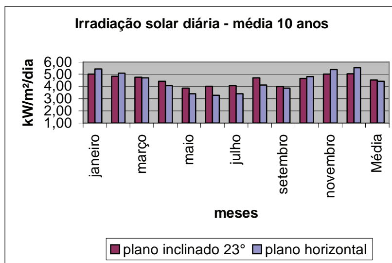
Figura 22. Irradiação solar diária para São Paulo, média de 10 anos, para o plano horizontal e para uma inclinação de 23° em relação ao Equador.
