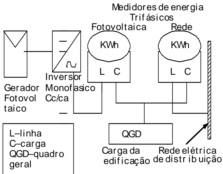
Figura 20. Diagrama unifilar dos medidores de energia e alimentação da carga.
