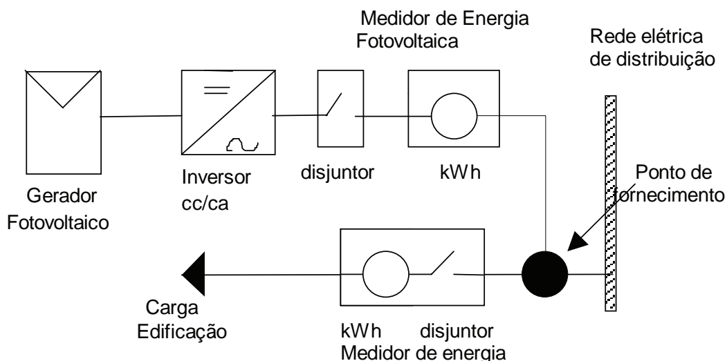
Figura 8. Esquema com Interconexão antes da medição – adaptado.
