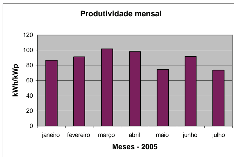
Figura 27. Produtividade mensal do sistema de 2,5 kWp.
