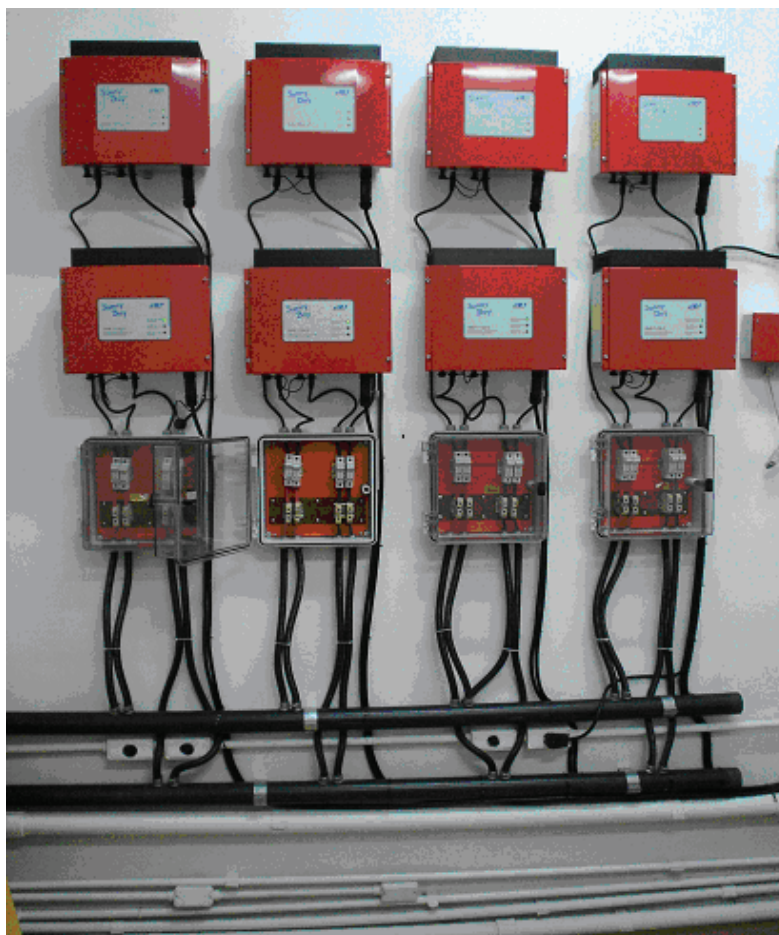
Figura 5. Instalação de inversores. A alimentação elétrica é em corrente contínua separada por pólo positivo e negativo em eletrodutos diferentes.
