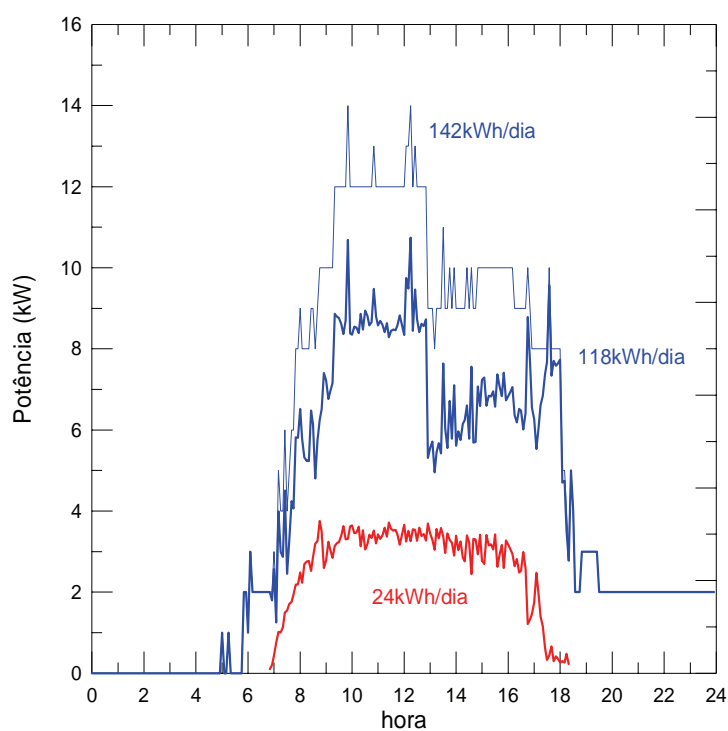
Figura 4. Curva de carga de prédio comercial com o consumo de energia (azul traço fino), energia fotogerada (em vermelho) e energia comprada da concessionária (azul traço grosso).
