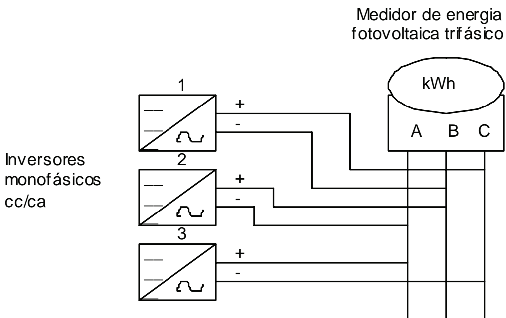
Figura 19. Esquema da ligação inversores monofásicos e medidor trifásico.
